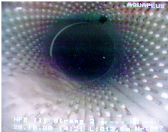
Untersuchung eines Horistranges mit Sandablagerungen
